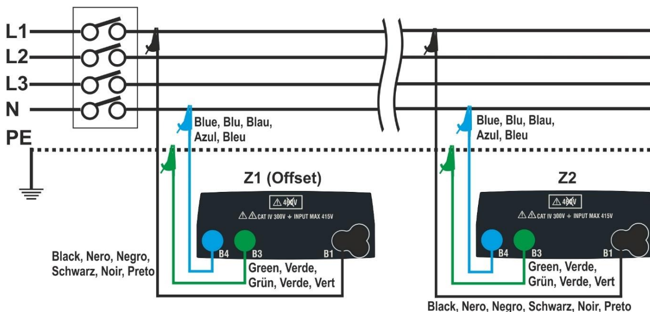
Fig.33: Tilslutning for måling af L-N-spændingsfald
