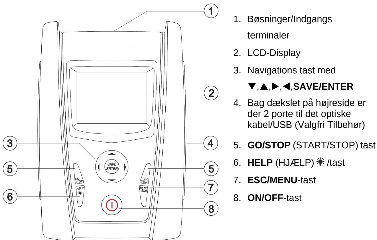
Fig 1 Beskrivelse af instrumentets front
