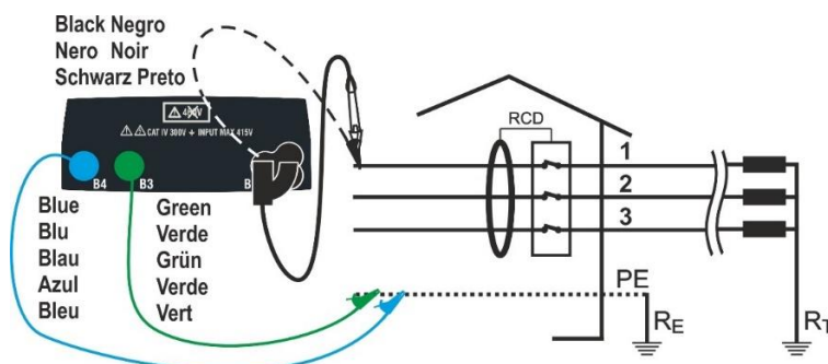
Fig. 21: 400V + PE (uden N) system med prøveledninger og fjernbetjeningsprobe
