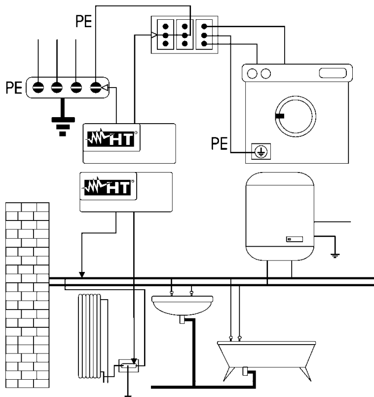
Fig.35 Eksempler på kontinuitetsmålinger på lederne
