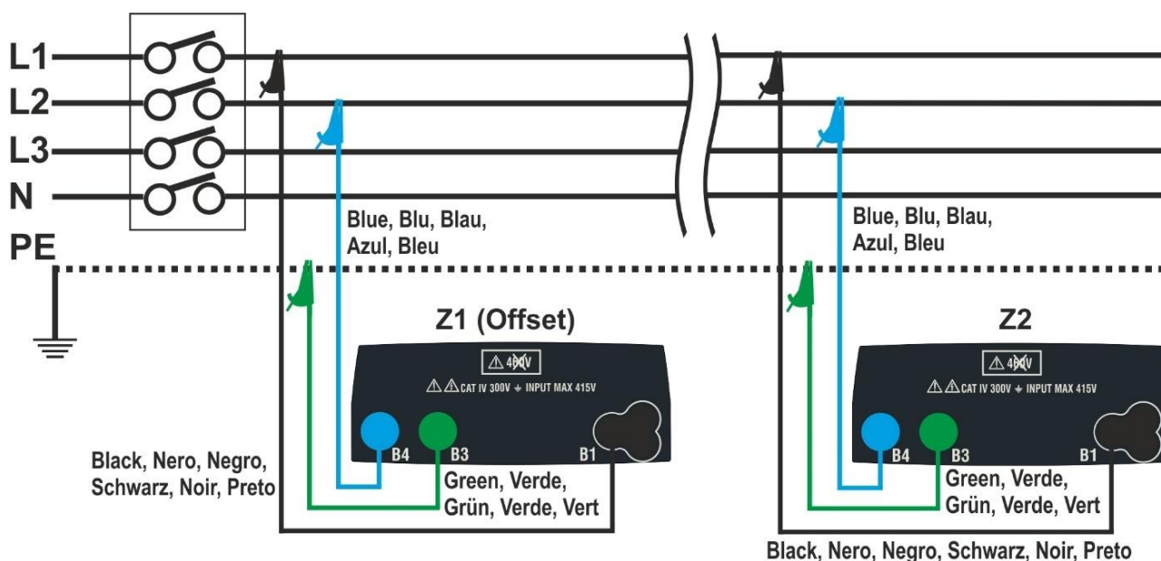
Fig. 34: Tilslutning for måling af L-L-spændingsfald
