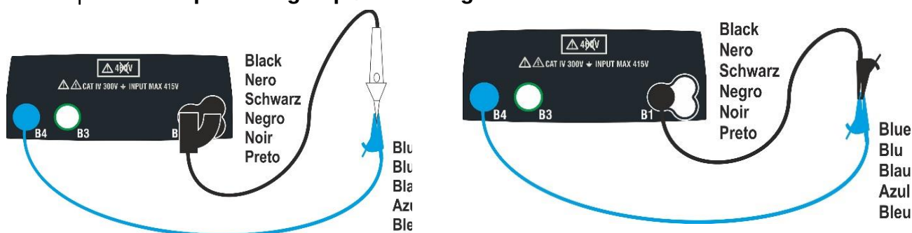
Fig. 10: Udkompensation af modstanden i prøveledning / i fjernbetjeningsproben
