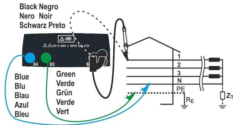
Fig.27: P-PE-måling på IT-systemer med prøveledninger og fjernbetjeningsprobe
